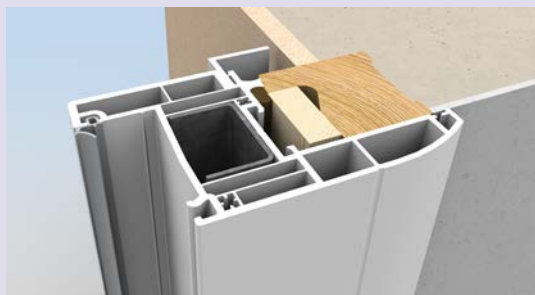
Rénovation avec aile de recouvrement monobloc de 60 mm.
