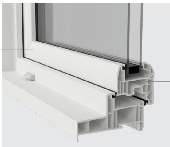
Profil ouvrant de 72 mm en forme contemporaine
