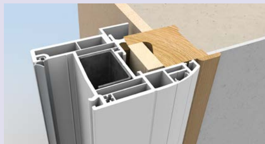
Rénovation avec aile de recouvrement monobloc de 40 mm.
