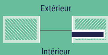
1 VANTAIL - 1 RAIL Refoulement à droite
